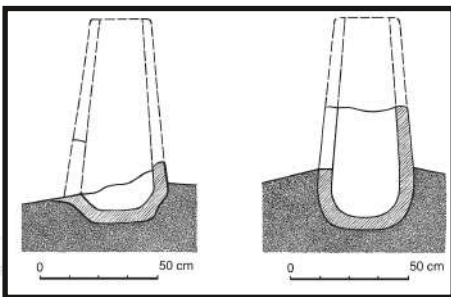
Řez typickou nadzemní šachtovitou pecí s mírně a kotlovitě zahluobenou nístějí.
